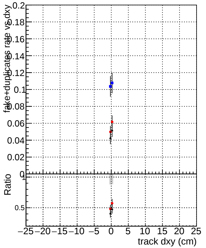
Legend: DQMstep3_TT_CKF DQMstep3_TT_default DQMstep3_TT_defaultNEWT20
