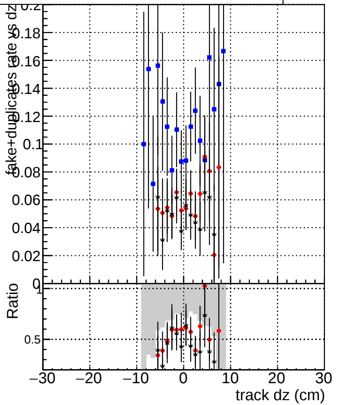
Legend: DQMstep3_TT_CKF DQMstep3_TT_default DQMstep3_TT_defaultNEWT20
