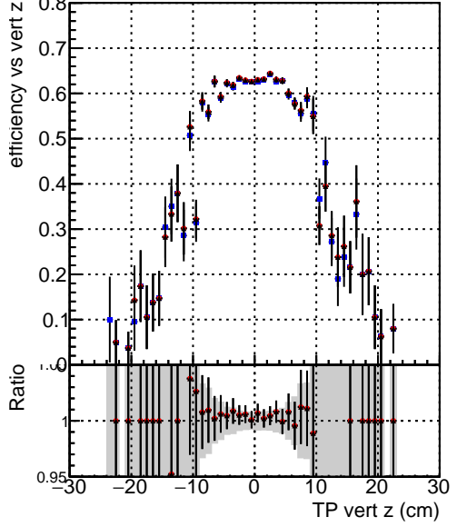
Efficiency vs. TP vert z —●— DQMstep3_TT_CKF —●— DQMstep3_TT_default —●— DQMstep3_TT_defaultNEWT20
