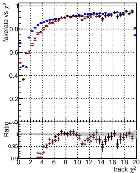
Fake rate vs. DOMstep3 TT GKF DOMstep3 default DOMstep3 defaultNEWT20
