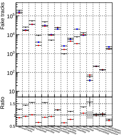
Number —●— DQMstep3_TT_default —▲— DQMstep3_TT_defaultNEWT20
