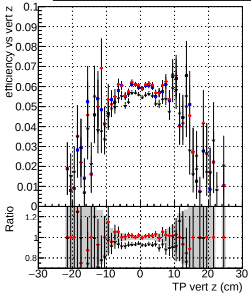
Efficiency vs. TP vert z (cm) —●— DQMstep3_TT_CKF —●— DQMstep3_TT_default —●— DQMstep3_TT_defaultNEWT20
