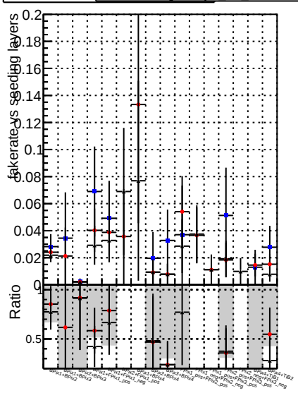
Fake rate vs. DOMstep3 CKF DOMstep3 default DOMstep3 default NEWT20
