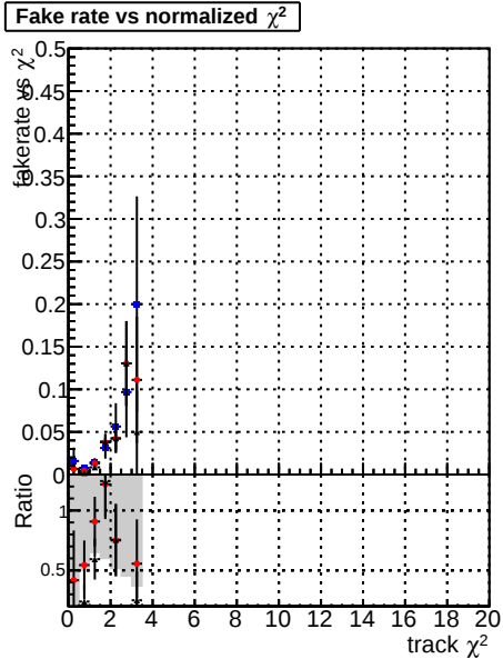
Fake rate vs. DOMstep3 CKF DOMstep3 default DOMstep3 default NEWT20
