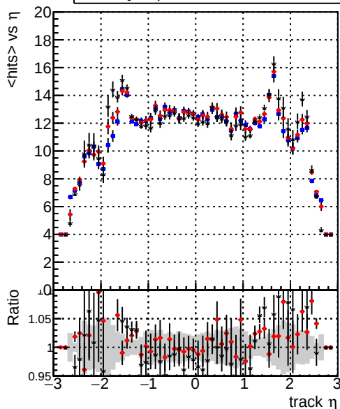
mean hit — DQMstep3_TT_CKF — DQMstep3_TT_default — DQMstep3_TT_defaultNEWT20
