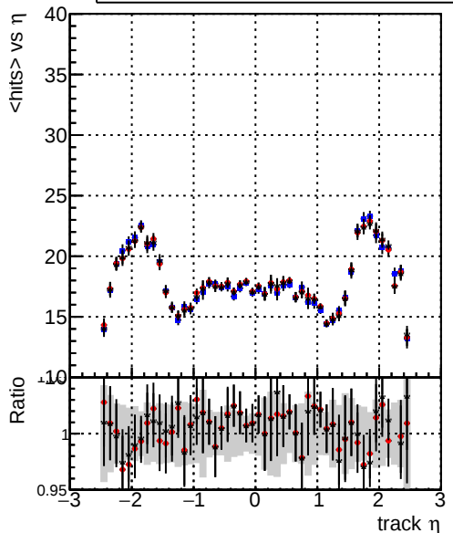
mean hits — DQMstep3_TT_CKF — DQMstep3_TT_default — DQMstep3_TT_defaultNEWT20
