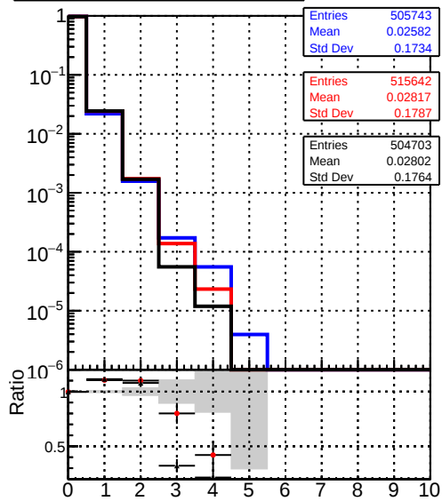
mean hits — DQMstep3_TT_CKF — DQMstep3_TT_default — DQMstep3_TT_defaultNEWT20
