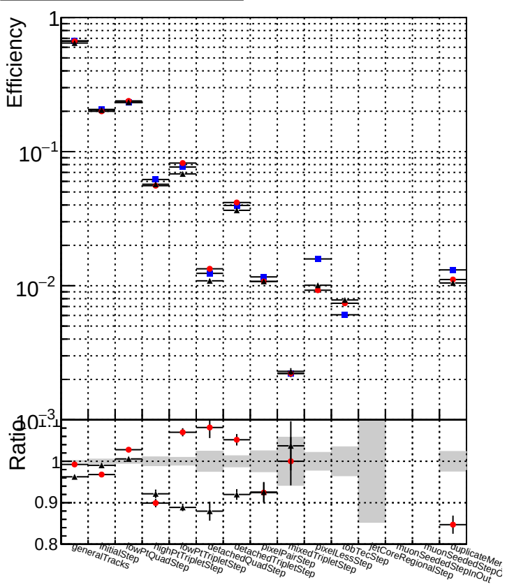
DQMstep3_TT_CKF DQMstep3_TT_default DQMstep3_TT_defaultNEWTreweight
