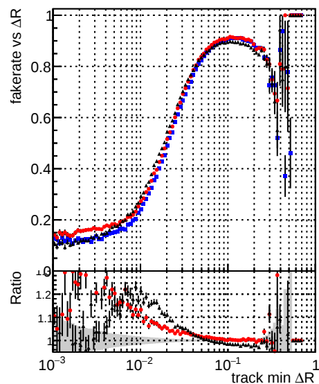
Legend: DQMstep3 TT CKF DQMstep3 TT default DQMstep3 TT defaultNEWTreweight
