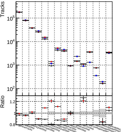
Number —■— DQMstep3_TT_CKF —●— DQMstep3_TT_default —▲— DQMstep3_TT_defaultNEWTweight
