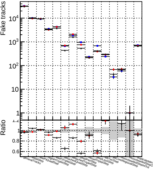
Number —■— DQMstep3_TT_CKF —●— DQMstep3_TT_default —▲— DQMstep3_TT_defaultNEWTweight
