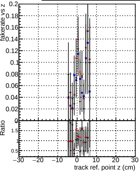
Fake rate vs verpos DOMstep3_TT_CKF DOMstep3_TT_default DOMstep3_TT_defaultNEWTweight
