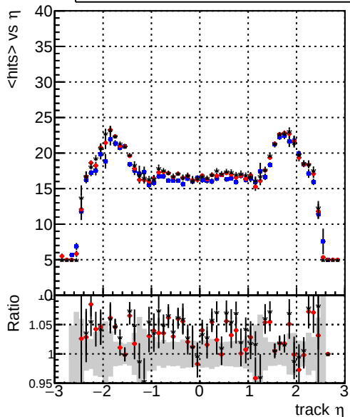
mean hits — DQMstep3_TT_CKF — DQMstep3_TT_default — DQMstep3_TT_defaultNEWTreweight
