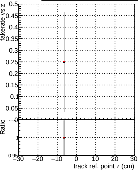
DOMstep3_TT_CKF DOMstep3_TT_default DOMstep3_TT_defaultNEWTreweight
