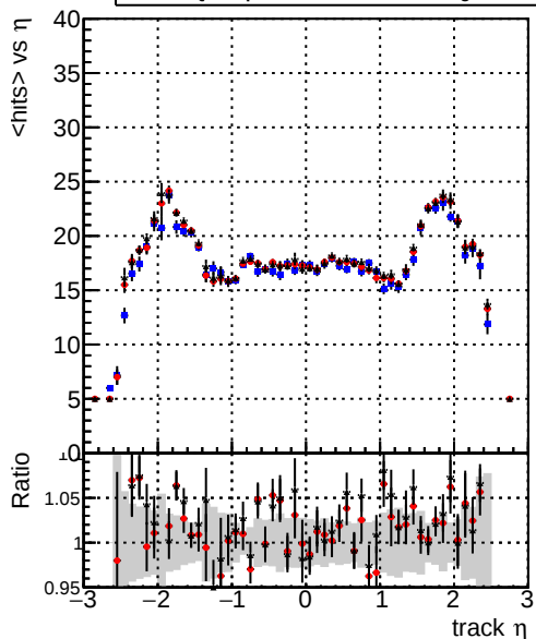
— DQMstep3_TT_CKF — DQMstep3_TT_default — DQMstep3_TT_defaultNEWTreweight mean hits
