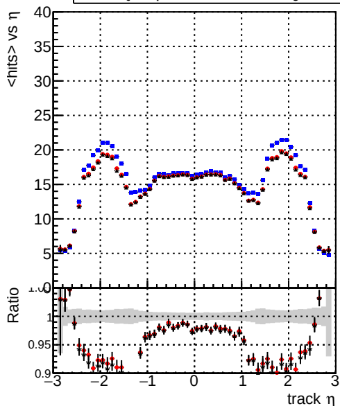
mean hits vs \eta — DQMstep3_TT_CKF — DQMstep3_TT_default — DQMstep3_TT_defaultNEWTreweight
