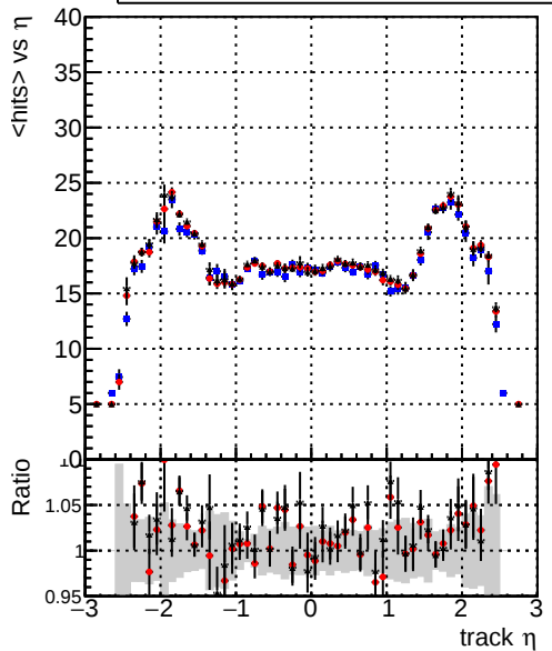
mean hit — DQMstep3_TT_CKF — DQMstep3_TT_default — DQMstep3_TT_defaultNEWTreweight
