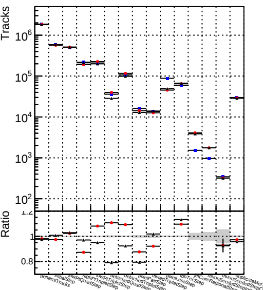
Number DQMstep3_TT_CKF DQMstep3_TT_default DQMstep3_TT_defaultNEWTreweight
