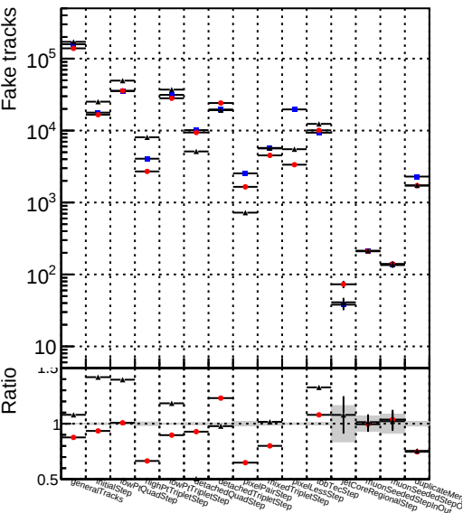
Number DQMstep3_TT_CKF DQMstep3_TT_default DQMstep3_TT_defaultNEWTreweight
