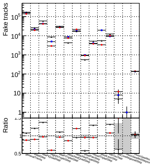
Number 1 ● DQMstep3_TT_default 2 ▲ DQMstep3_TT_defaultNEWTreweight
