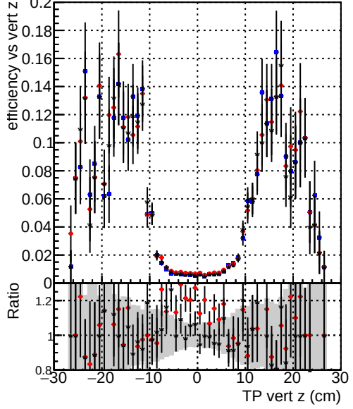
Efficiency vs. TP vert z (cm) —●— DQMstep3 TT_CKF —●— DQMstep3 TT_default —●— DQMstep3 TT_defaultNEWTreweight
