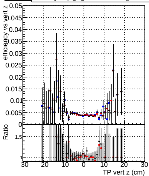
Efficiency vs. TP vert z (cm) Legend: - DQMstep3_TT_CKF (blue circles) - DQMstep3_TT_default (red circles) - DQMstep3_TT_defaultNEWTreweight (black crosses)
