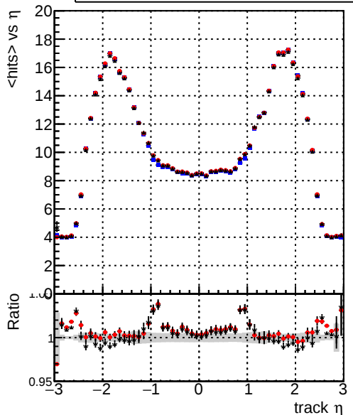
DQMstep3_TT_CKF DQMstep3_TT_default DQMstep3_TT_defaultNEWTreweight mean hits
