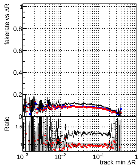
—●— DQMstep3_TT_CKF —●— DQMstep3_TT_default —●— DQMstep3_TT_defaultNEWTweight
