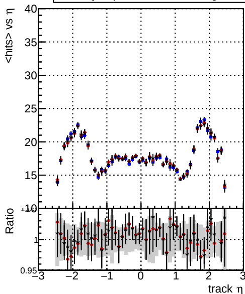
mean hits vs \eta — DQMstep3_TT_CKF — DQMstep3_TT_default — DQMstep3_TT_defaultNEWTreweight
