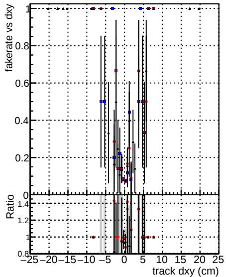
— DOMstep3 TT CKF — DOMstep3 TT default — DOMstep3 TT defaultNEWtreweight
