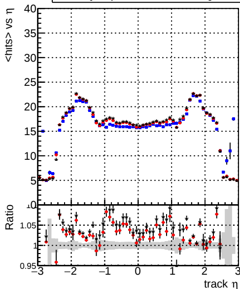
— DQMstep3_TT_CKF — DQMstep3_TT_default — DQMstep3_TT_defaultNEWTreweight mean hits
