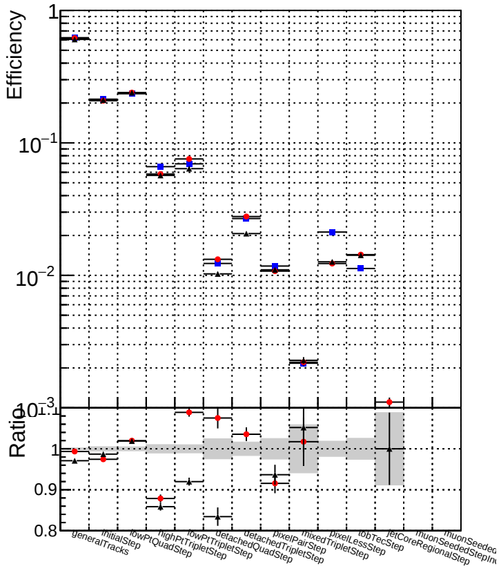
DQMStep3_TT_CKF DQMStep3_TT_default DQMStep3_TT_defaultNEWT-oldsamples
