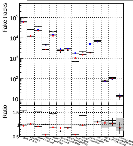
Number Legend 1 DQMstep3_TT_default 2 DQMstep3_TT_default+NEWTON-oldsamples
