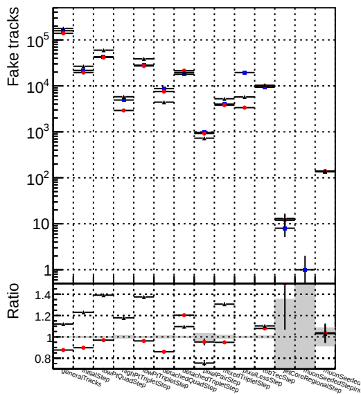
Number Legend —●— DQMstep3_TT_default —▲— DQMstep3_TT_defaultNEWT-oldsamples
