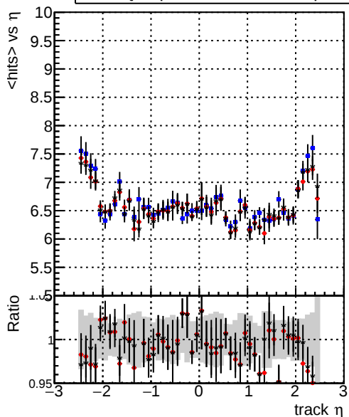
mean hits vs \eta Legend: DQMstep3_TT_CKF (blue), DQMstep3_TT_default (red), DQMstep3_TT_defaultNEWT-oldsamples (black)
