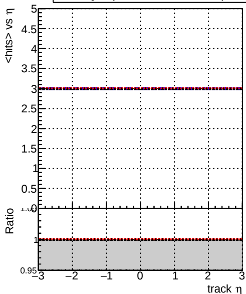
mean hits — DQMstep3_TT_CKF — DQMstep3_TT_default — DQMstep3_TT_defaultNEWT-oldsamples
