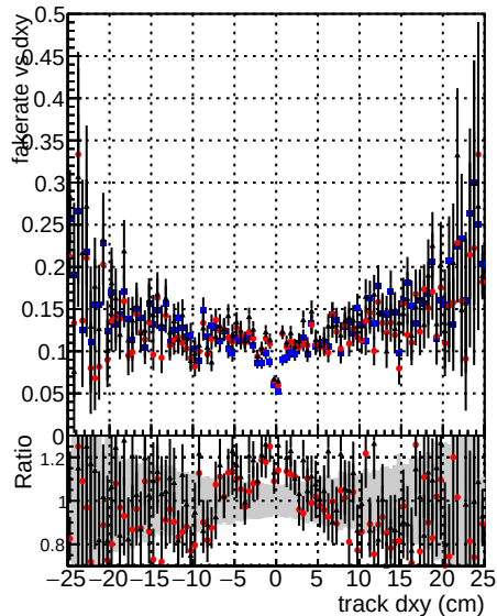
—●— DOMstep3 TT CKF —●— DOMstep3 default —●— default NEWT-oldsamples
