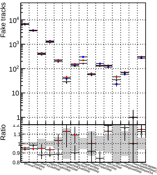
Number Legend ● DQMstep3_TT_default ▲ DQMstep3_TT_defaultNEWT-oldsamples
