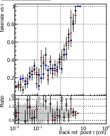
Fake rate vs v —●— DQMstep3 TT CKF —●— DQMstep3 TT default —●— DQMstep3 TT defaultNEWT-oldsamples
