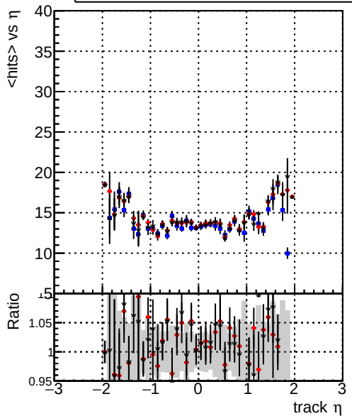
mean hit — DQMstep3_TT_CKF — DQMstep3_TT_default — DQMstep3_TT_defaultNEWT-oldsamples
