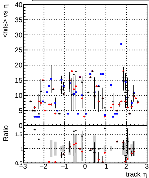
— DQMstep3_TT_CKF — DQMstep3_TT_default — DQMstep3_TT_defaultNEWT-oldsamples mean hits
