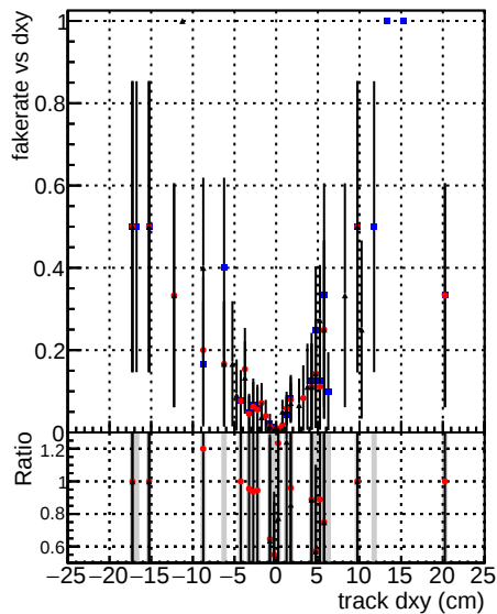
—•— DOMstep3 TT CKF —•— DOMstep3 TT default —•— DOMstep3 TT defaultNEWT-oldsamples
