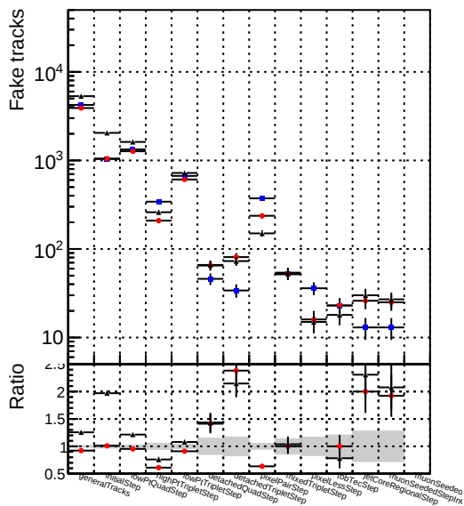
Number of tracks vs collection Legend: DQMstep3_TT_CKF DQMstep3_TT_default DQMstep3_TT_defaultNEWT-oldsamples
