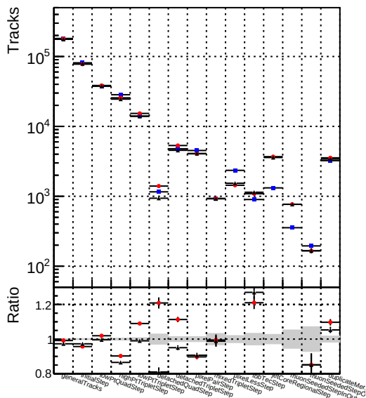
DQMstep3_TT_CKF DQMstep3_TT_default DQMstep3_TT_defaultNEW-oldsamples
