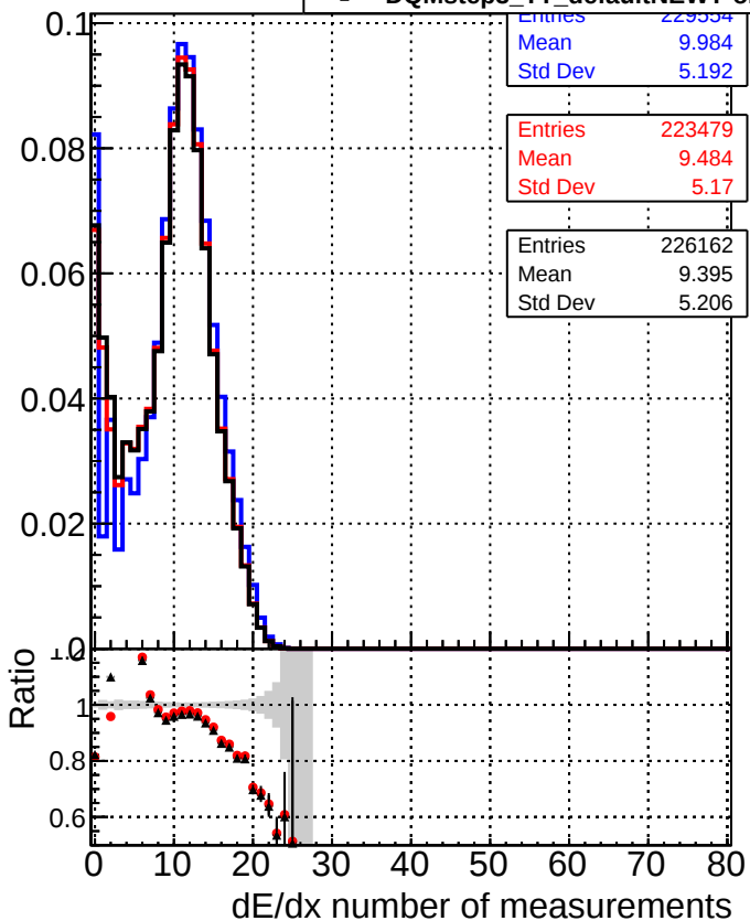
Legend: —■— DQMstep3_TT_CKF —●— DQMstep3_TT_default —▲— DQMstep3_TT_defaultNEWT-oldsamples
