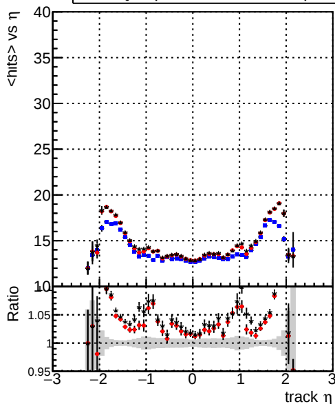
mean hits vs \eta — DQMstep3_TT_CKF — DQMstep3_TT_default — DQMstep3_TT_defaultNEWT-oldsamples
