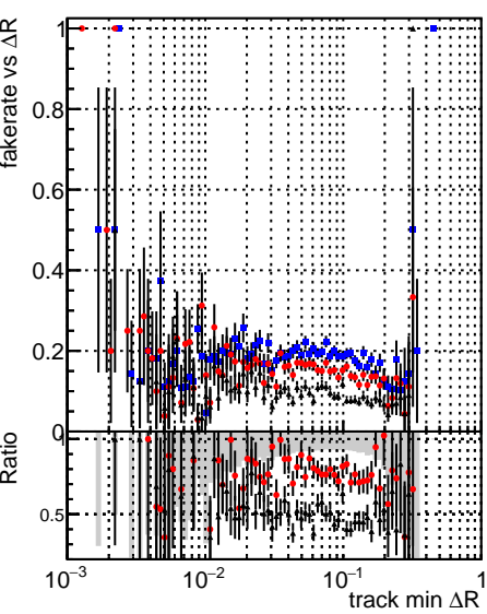
■ DQMstep3_TT_CKF ● DQMstep3_TT_default + DQMstep3_TT_defaultNEWT-oldsamples
