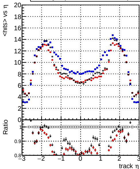
— DQMstep3_TT_CKF — DQMstep3_TT_default — DQMstep3_TT_defaultNEWT-oldsamples mean hits
