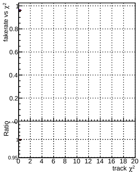
Fake rate vs. DOMstep3 TT CKF DOMstep3 TT default DOMstep3 TT defaultNEWTepo7
