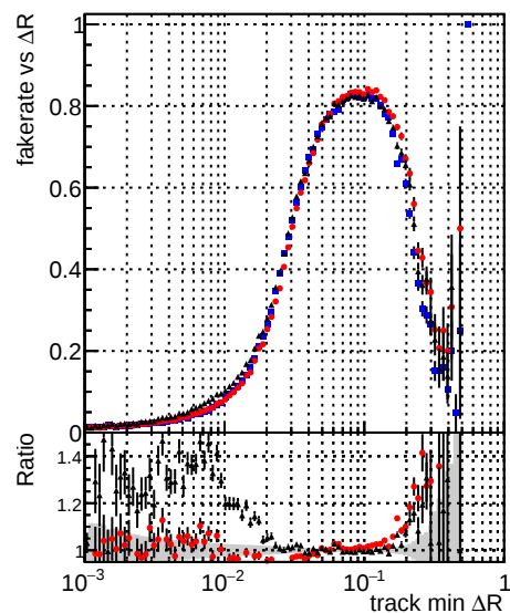
Legend: DQMstep3_TT_CKF (blue stars) DQMstep3_TT_default (red stars) DQMstep3_TT_defaultNEWTepo7 (black stars)
