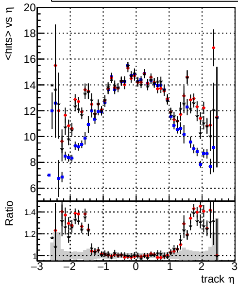
mean hits vs \eta — DQMstep3_TT_CKF — DQMstep3_TT_default — DQMstep3_TT_defaultNEWTepo7
