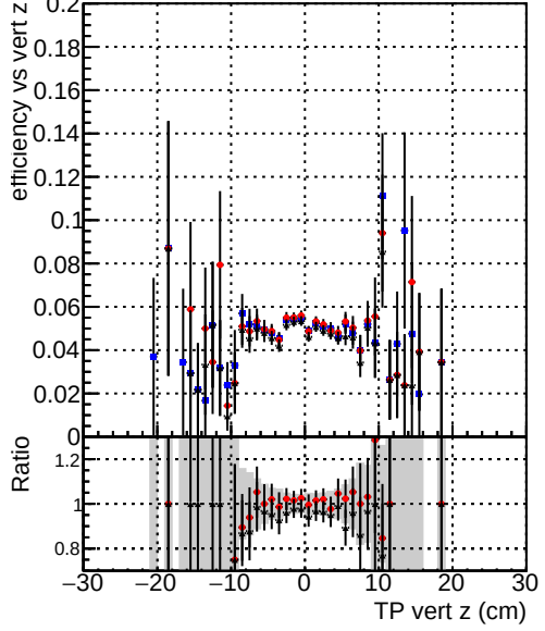
Efficiency vs. TP vert z (cm) —●— DQMstep3_TT_CKF —●— DQMstep3_TT_default —●— DQMstep3_TT_defaultNEWTepo7
