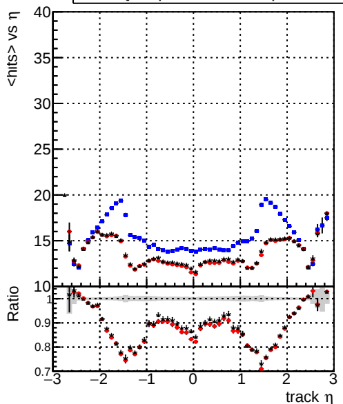
— DQMstep3_TT_CKF — DQMstep3_TT_default — DQMstep3_TT_defaultNEWTepo7 mean hits vs \eta
