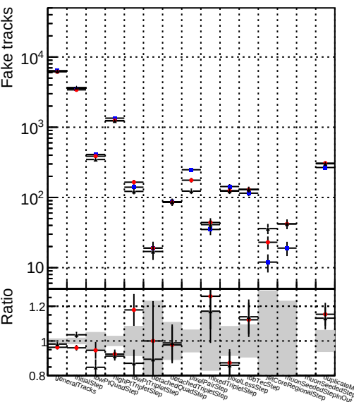
Number Series 1 DQMstep3_TT_default 2 DQMstep3_TT_defaultNEWTepo7
